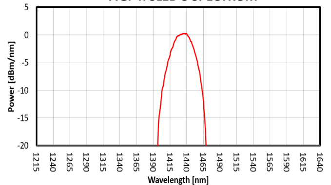
FIG. 4: SLED 3 SPECTRUM
