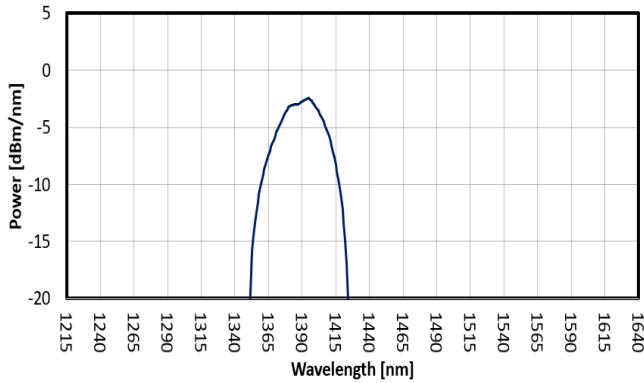
FIG. 7: SLED 6 SPECTRUM
