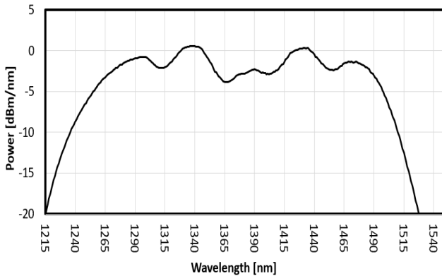
FIG. 1: ISB2 SPECTRUM
