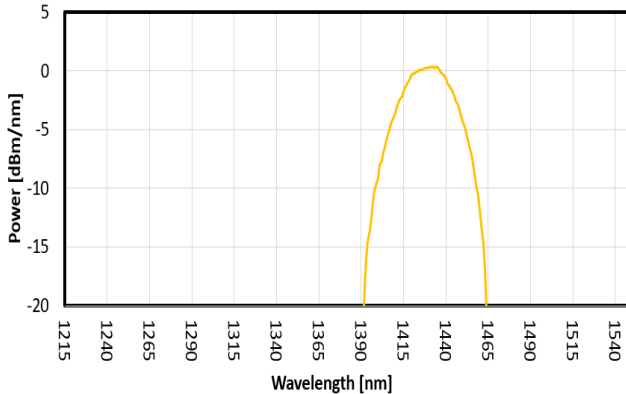
FIG. 3: SLED 2 SPECTRUM
