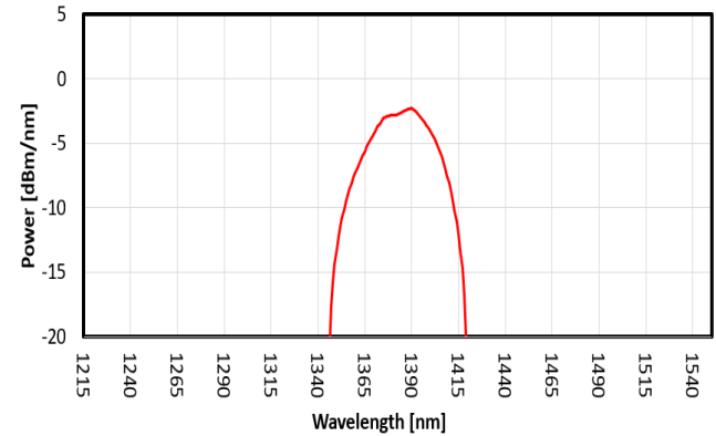
FIG. 4: SLED 3 SPECTRUM
