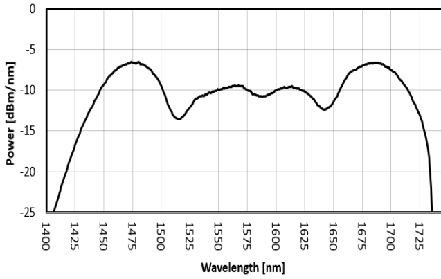
FIG. 1: ISB2 SPECTRUM
