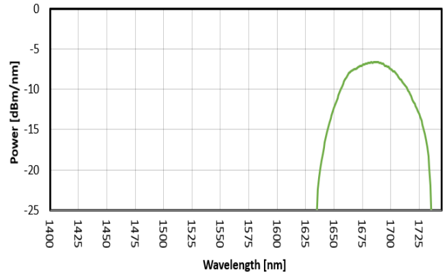
FIG. 2: SLED 1 SPECTRUM
