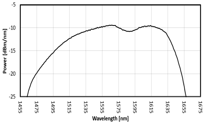
FIG. 1: OSE2 SPECTRUM
