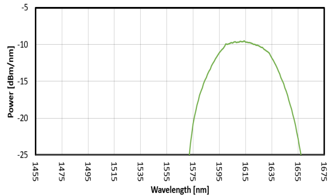
FIG. 2: SLED 1 SPECTRUM
