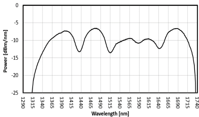
FIG. 1: OSE2 SPECTRUM
