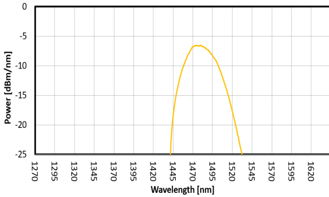
FIG. 3: SLED 2 SPECTRUM
