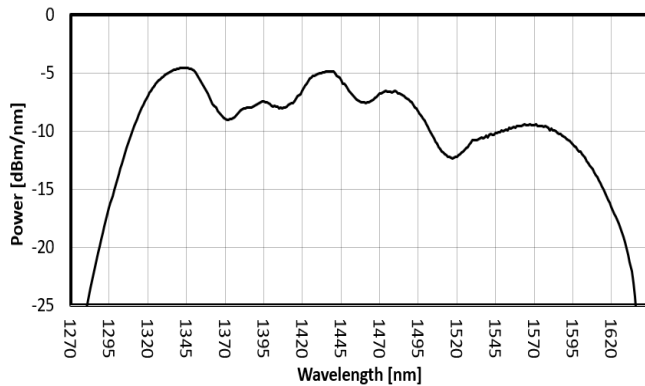
FIG. 1: OSE2 SPECTRUM
