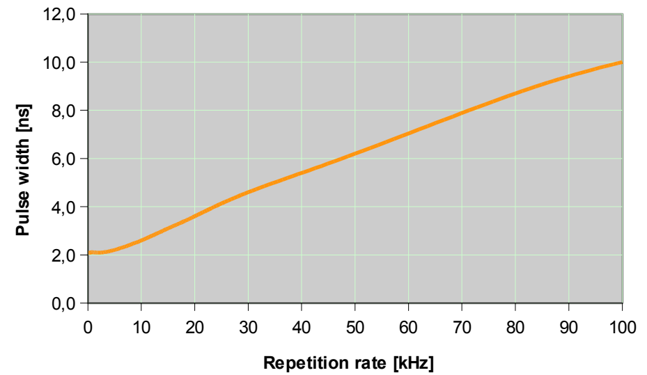
Onda 1064nm: Pulse Width
