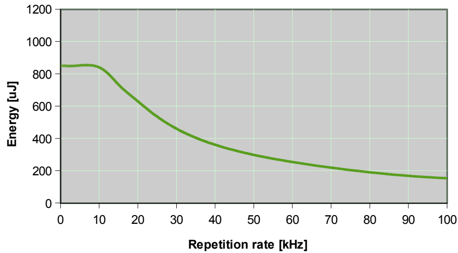
Onda 1064nm: Pulse Energy
